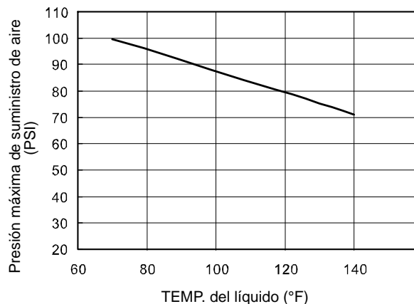
Curva de presión máxima de suministro de aire en función de la TEMPERATURA del líquido/líquido
